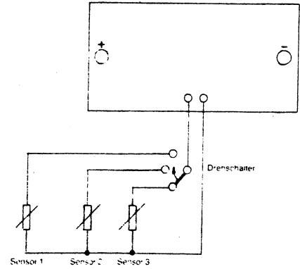
Schaltbeispiel für drei Meßstellen
