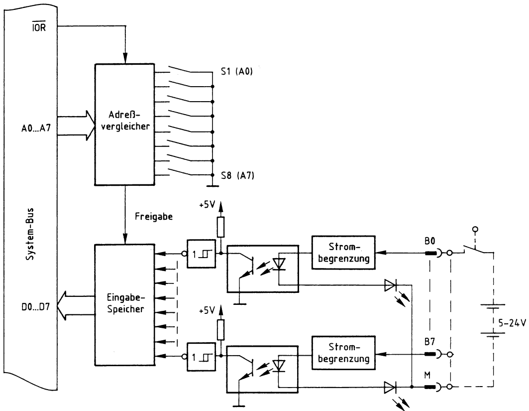
Bild 6: Das Blockschaltbild der 8-Bit-Parallel-Eingabe-Baugruppe mit galvanischer Trennung der Eingangs-Signale vom Mikrocomputer-System.
