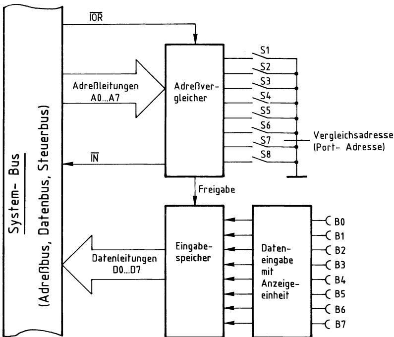
Bild 1: Blockschaltbild der Baugruppe »8-Bit-Parallel-Eingabe«.
