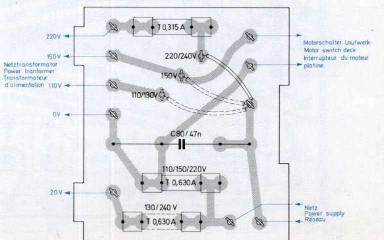
Fig. 9 Netzplatte 230 608 (Bestückungsseite)
