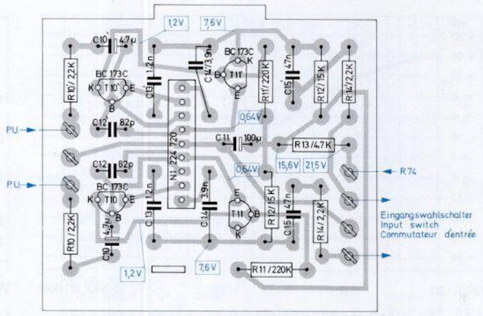
Fig. 7 Vorverstärker 227 585 (Leiterseite)
