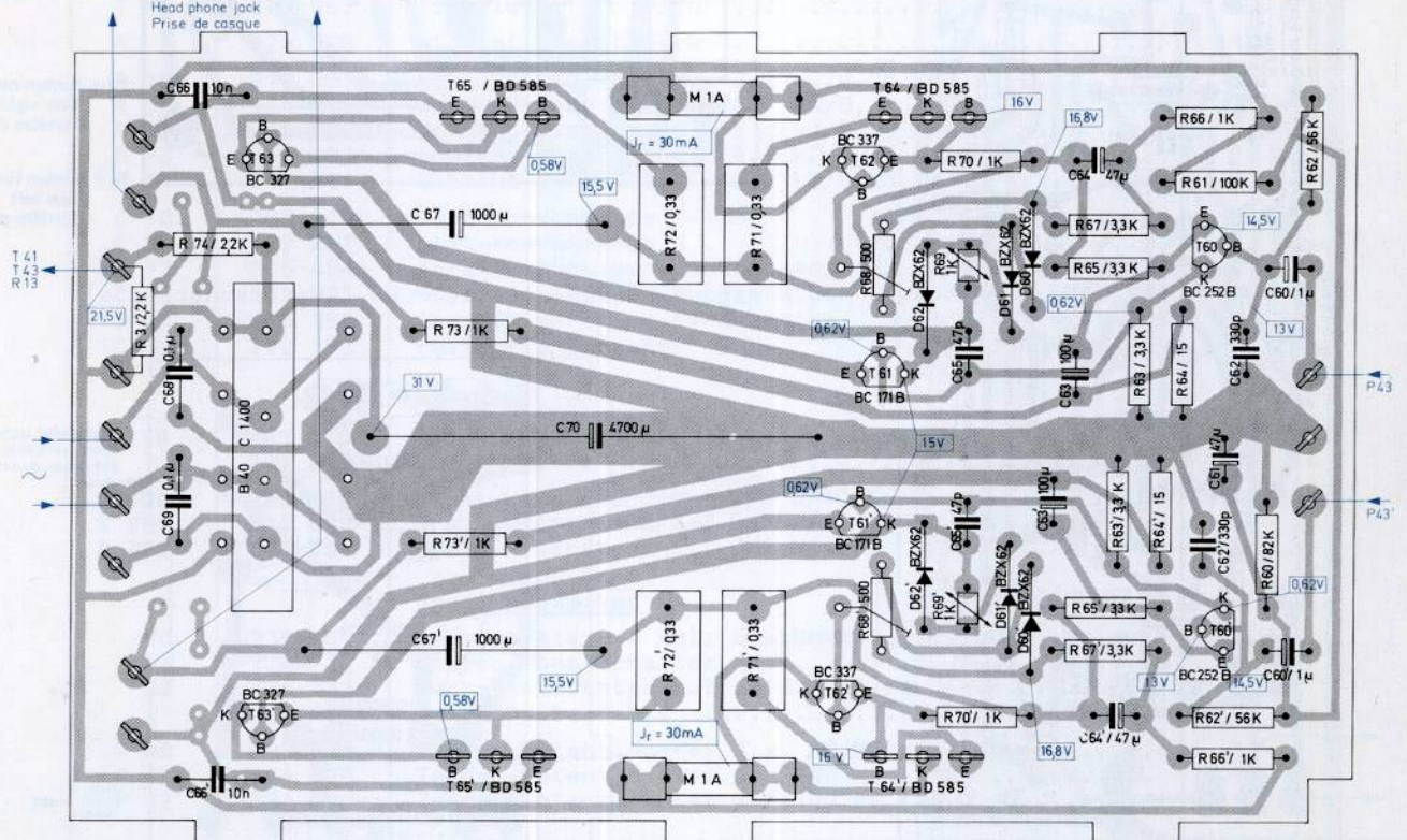
Fig. 5 Endverstärker 227 587 (Leiterseite)
